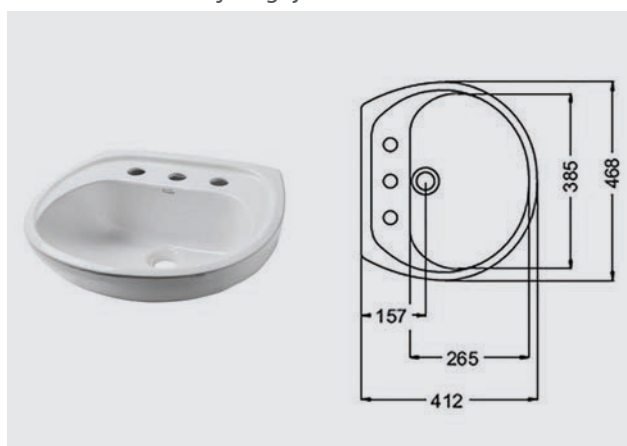
Andina lavatorio 3 y 1 agujeros
