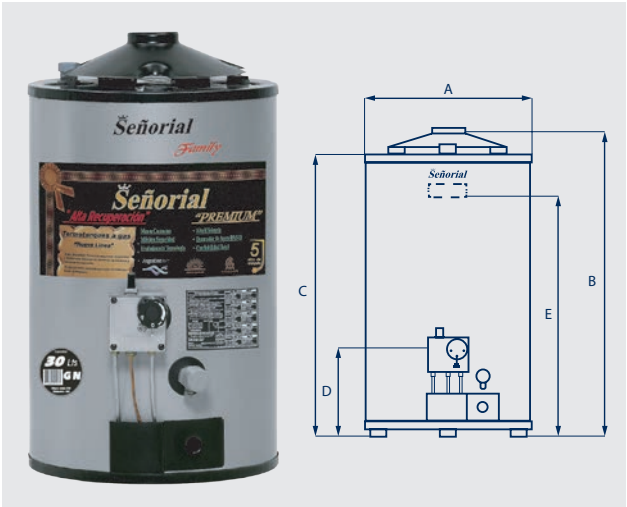
Termotanque Alta Recuperación Gris a Gas 30 y 50 Lts.
