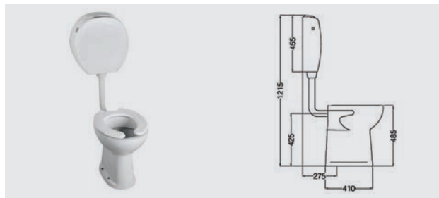
Inodoro para discapacitados IETI
