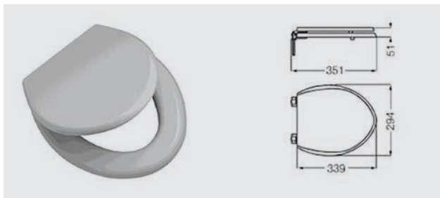
Tapa para inodoro para niños TCM
