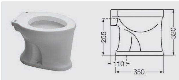
Inodoro para niños ICM
