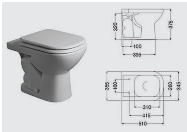
Bari IKCM-B: Inodoro corto
