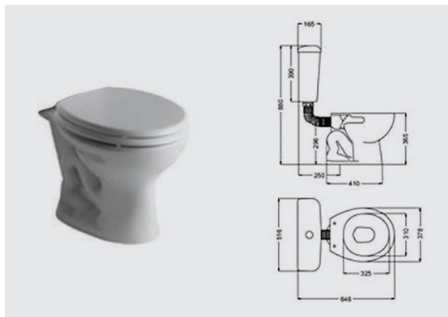
Andina IFA-B: inodoro corto
