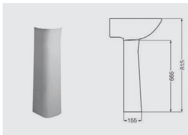
Bari CKC-B: Columna Blanca
