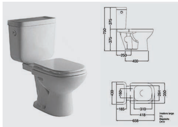
Bari IKLM-B: Inodoro Largo
