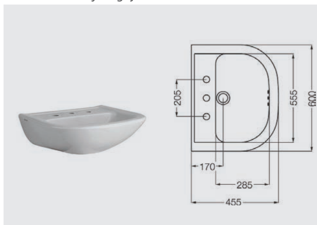
Bari lavatorio 3 y 1 agujero
