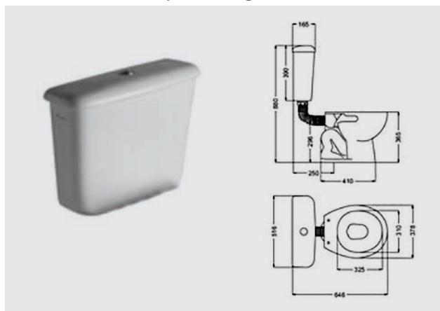
Andina DPCXF-B: depósito colgar
